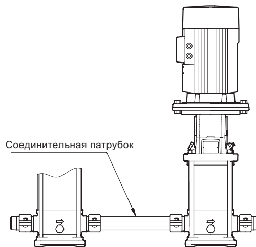
Рис. 32 Соединительный патрубок
