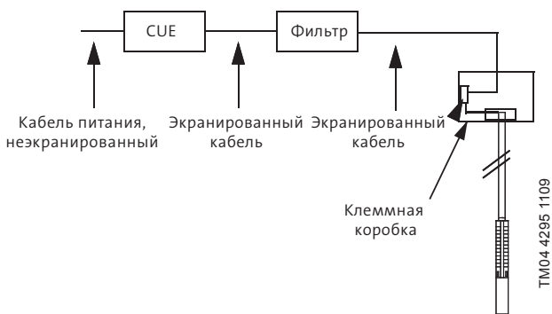
Рис. 3. Пример установки в зонах, чувствительных к радиопомехам
